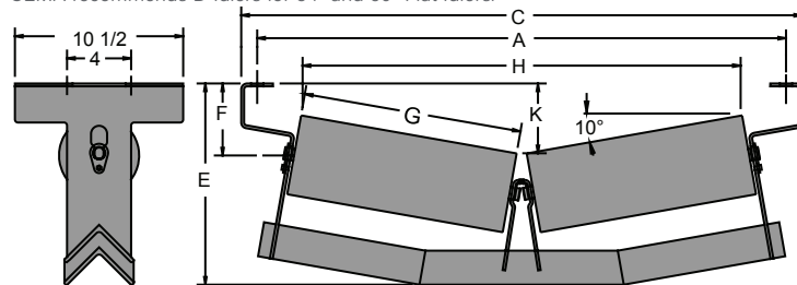
V-RETURN IDLER (F = 4 1/2")
